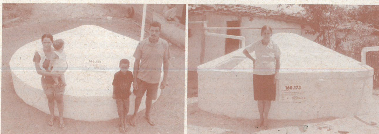
A construção da cisterna de placa reúne tecnologias sociais de baixo custo, oferecendo condições para armazenar 16 mil litros de água da chuva o que garante, para uma família de até cinco pessoas, o consumo por um período entre seis e oito meses. Outras tecnologias além das cisternas de placa, como barragens subterrâneas e cisternas calçadão, para produção básica de alimentos, também são experimentadas pelo programa.
